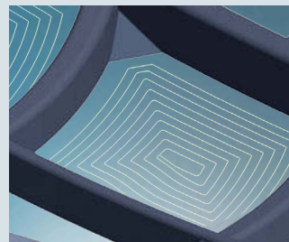
5軸シェイプ・オフセット仕上げ加工 の底面のみ
