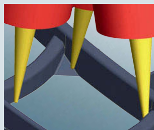
5軸スweep加工でのテーパボ ール仕上げ
