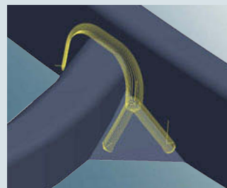
5軸削り残り部加工のオートマチック・インデックス
