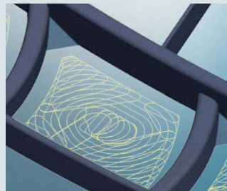
5軸シェイプ・オフセット荒加工 with hyperMAXX®：5軸トロコイド 加工を実現
