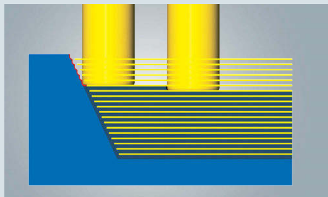
切り込み量を最小化した従来型の加工手法
