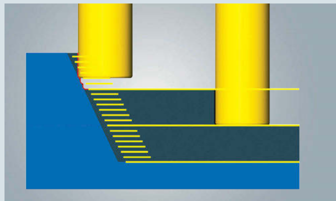
大きな切り込み量と中間ステップを使用した HPC 加工
