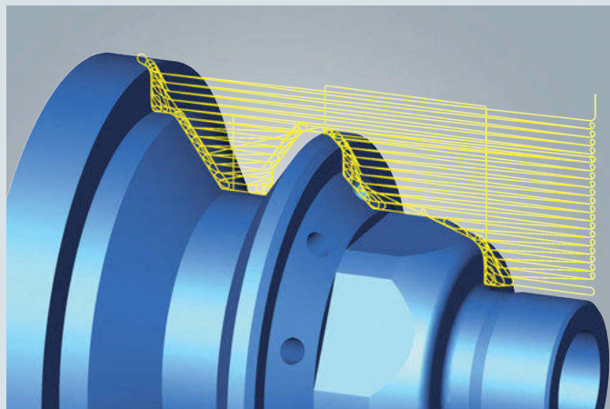
トロコイド状のツールパスによるハイパフォーマンス旋削加工
