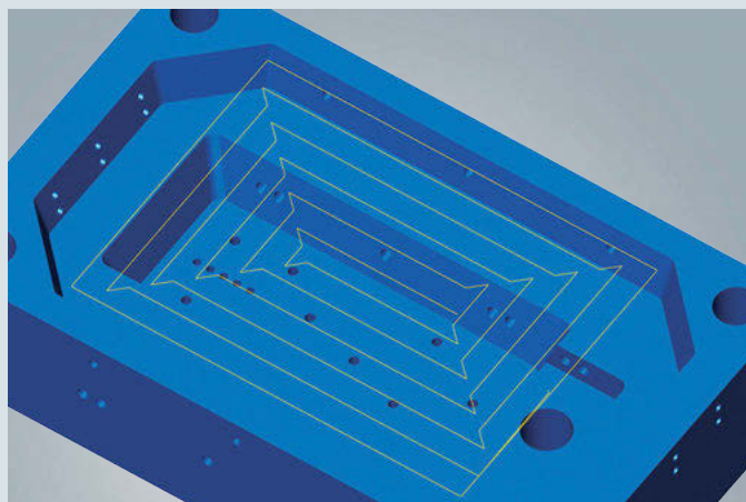
高送り加工を最適化したポケット加工
