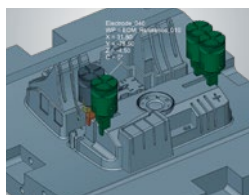
Виртуальный электрод
