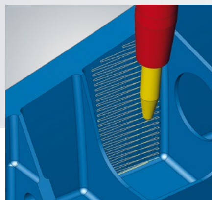
5-осевая тангенциальная обработка поверхностей
